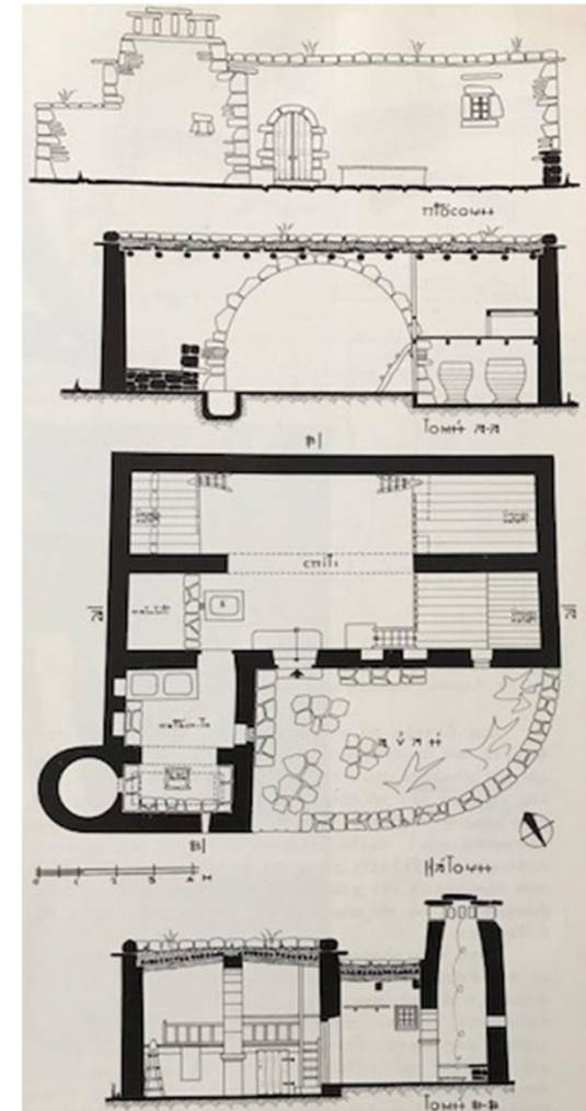
σχέδια από το καμαρόσπιτο
