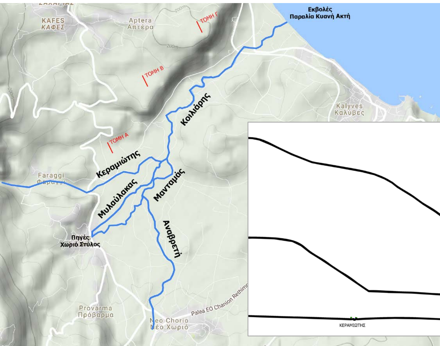
Τομές ανάγλυφου κατά μήκος του ποταμού
