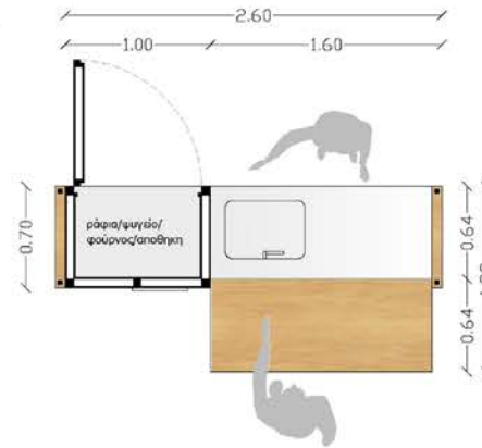
ΚΑΤΟΨΗ
