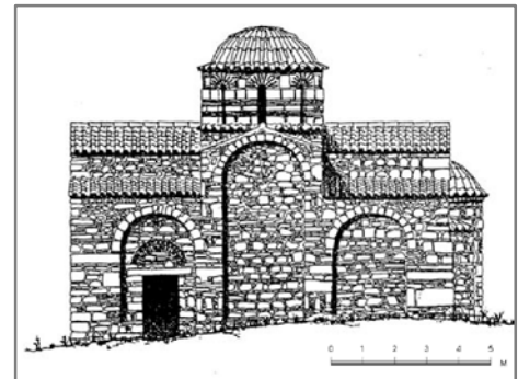
Νότια όψη
