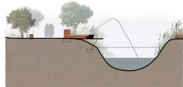
τομή εγκατάστασης για ερασιτεχνική αλιεία
