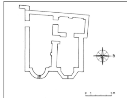
Κάτοψη
