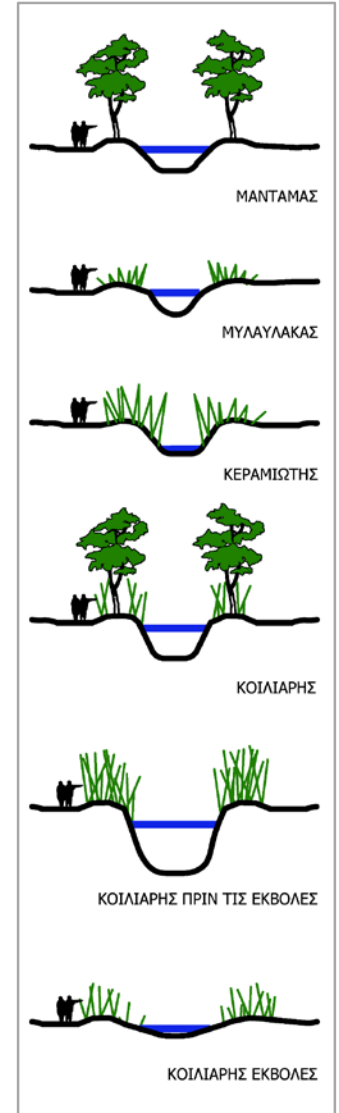
Τομές Κοιλίερη και παραπόταμων με παρόχθια βλάστηση
