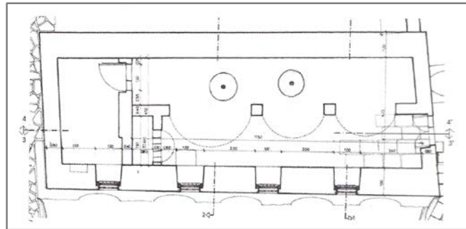
Κάτοψη
