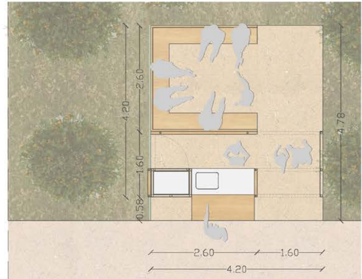
Διαμόρφωση εισόδου σε εκπαιδευτικά αγροκτήματα - Κάτοψη
