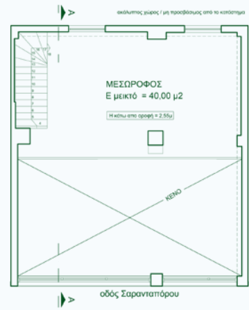
ΚΑΤΟΨΗ ΜΕΣΩΡΟΦΟΥ
