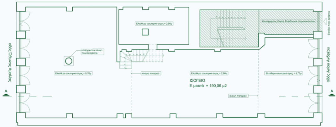
ΧΩΡΟΣ Α, ΥΠΑΡΧΟΥΣΑ ΚΑΤΑΣΤΑΣΗ, ΚΑΤΟΨΗ ΙΣΟΓΕΙΟΥ
