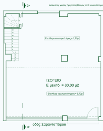
ΧΩΡΟΣ Β, ΥΠΑΡΧΟΥΣΑ ΚΑΤΑΣΤΑΣΗ, ΚΑΤΟΨΗ ΙΣΟΓΕΙΟΥ
